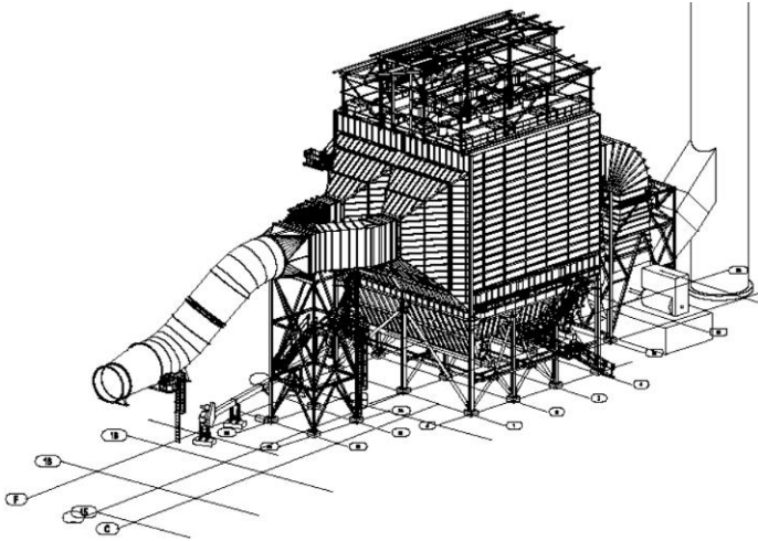
Precipitador electrostático y conducto de entrada planta SINTER
