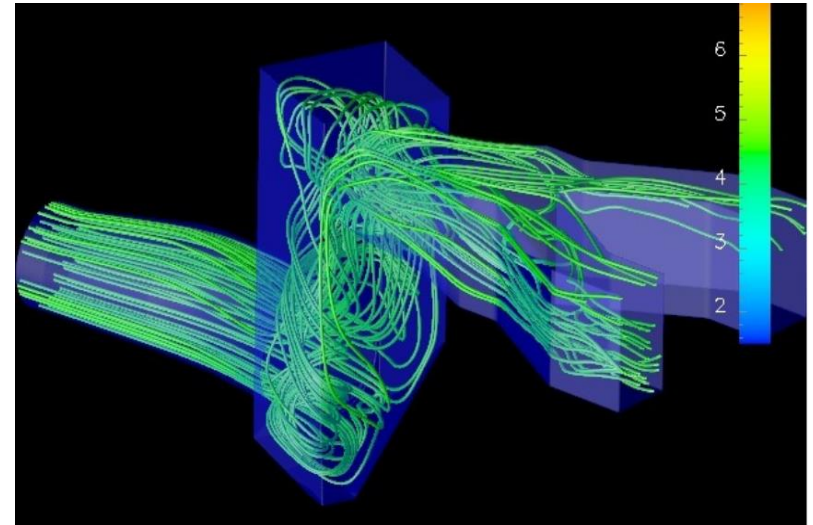
Patrón de flujo en la manga de entrada al precipitador
